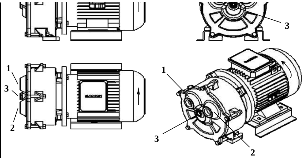
Şekil - 21 : PVM serisi tasarım tipi C
