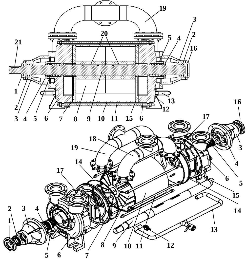
Şekil-35 : PVN Serisi B Tip Vakum Pompaları
