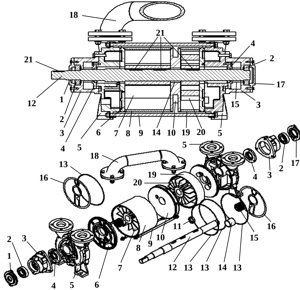
Şekil-34 : PVN Serisi A Tip Vakum Pompaları
