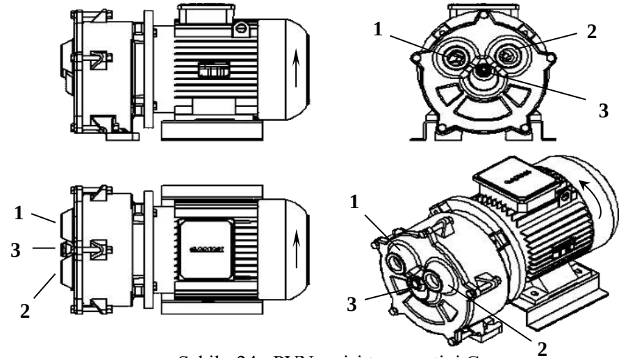
Şekil - 24 : PVN serisi tasarım tipi C
