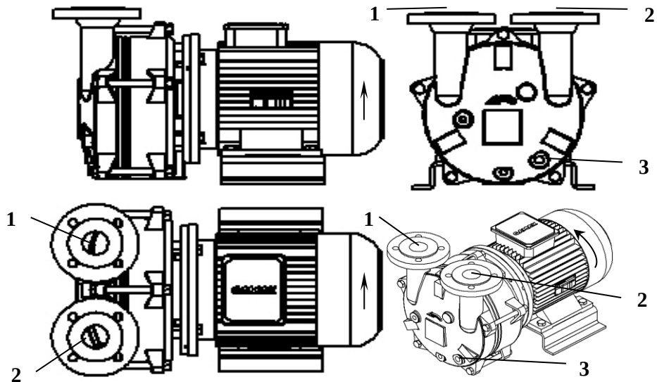
Şekil - 22 : PVN serisi tasarım tipi A
