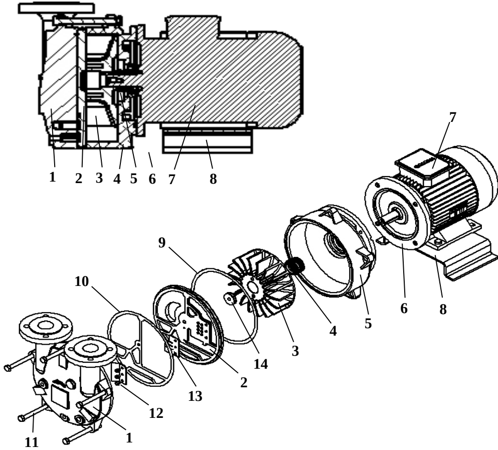
Şekil-32 : PVM Serisi A Tip Vakum Pompaları
