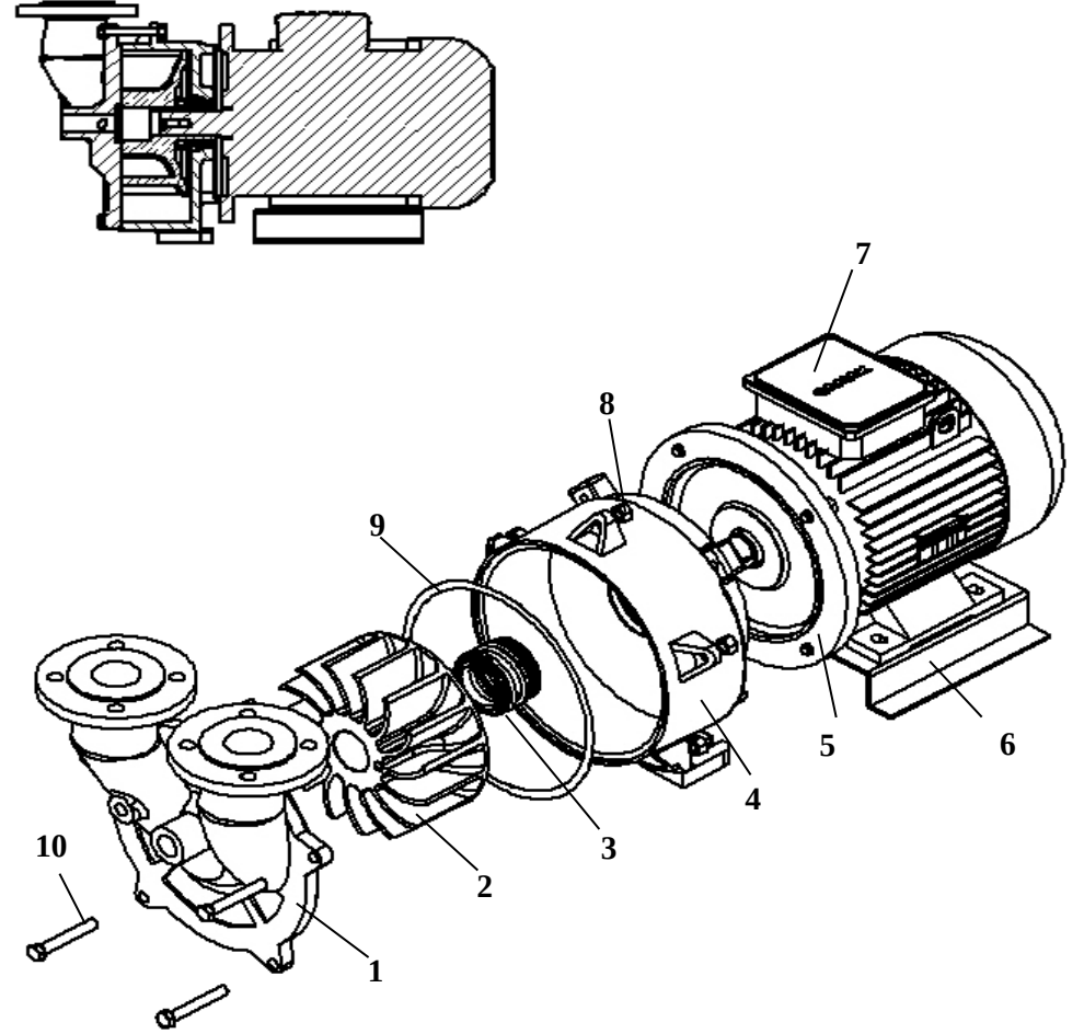
Şekil-33 : PVM Serisi B Tip Vakum Pompaları
